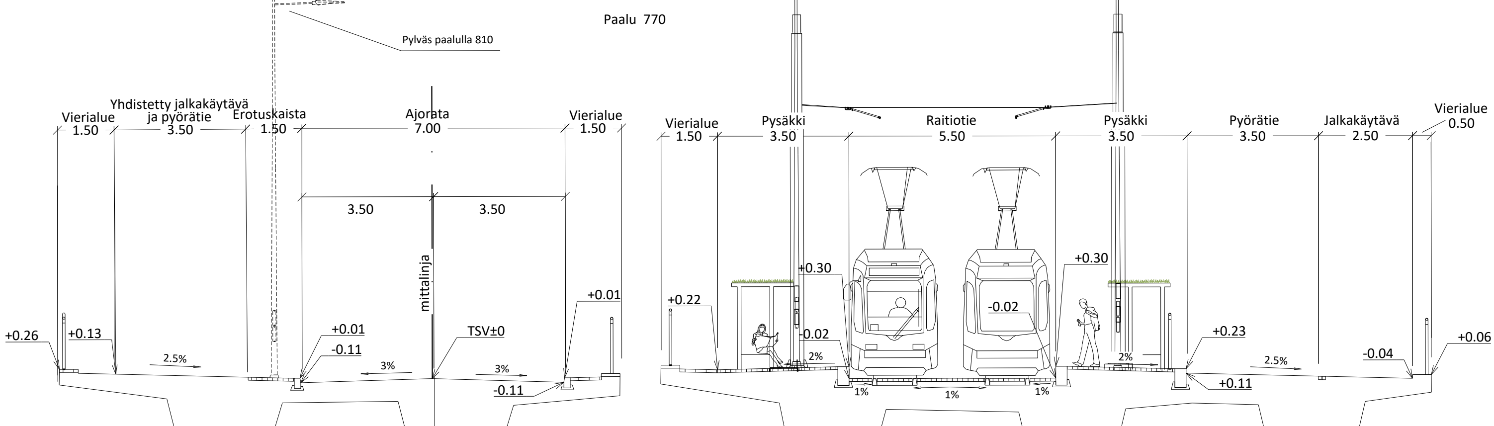
Tyyppipoikkileikkaus F-F
