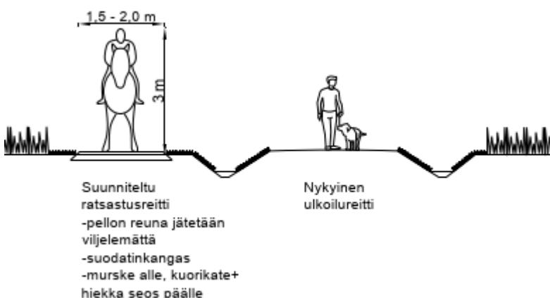
Kuva 1. Periaateleikkaus suunnitellusta ratsastusreitistä pellon reunaan nykyisen ulkoilureitin viereen.
